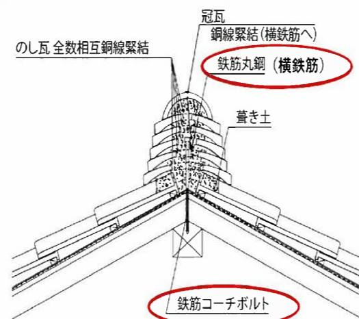
耐震工法・断面図
