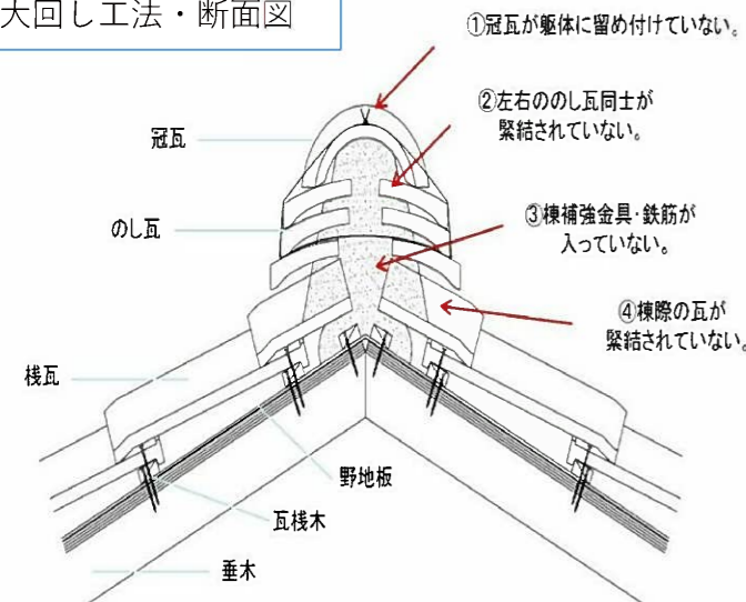
大回し工法・断面図
